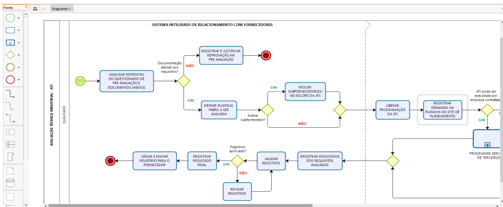
FIGURA 6 – Mapa do subprocesso de ATI (Visão Parcial)
