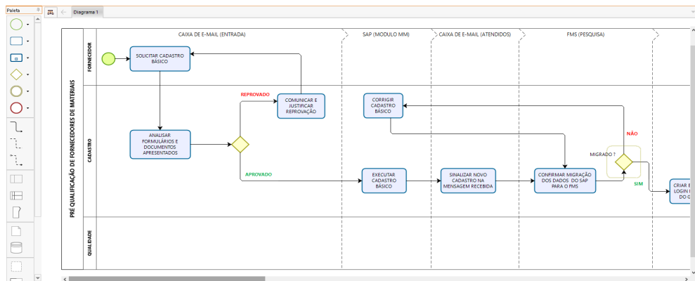
FIGURA 3 – Mapa do processo de pré-qualificação de fornecedores de materiais da empresa Energia (Visão Parcial)
