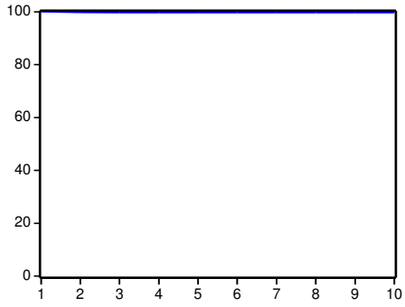
Percentual da variancia de RIBOV devido a RIBOV
