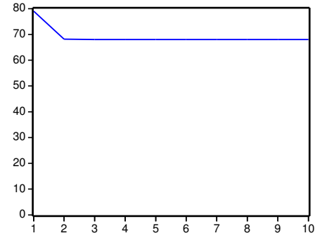
Percentual da variancia de RRTS devido a RRTS
