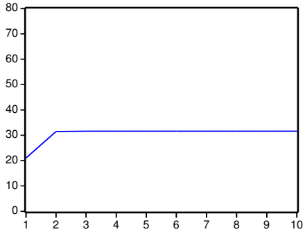
Percentual da variancia de RRTS devido a RIBOV
