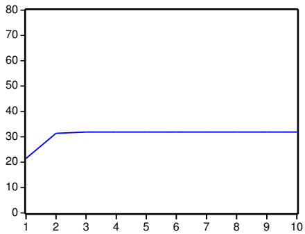
Percentual da variancia de RHS devido a RIBOV
