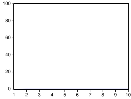
Percentual da variancia de RIBOV devido a RRTS
