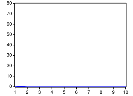
Percentual da variancia de RRTS devido a RHS
