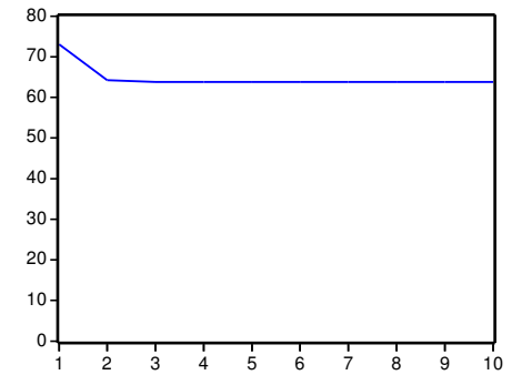
Percentual da variancia de RHS devido a RHS
