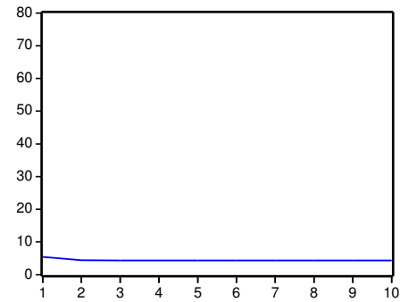
Percentual da variancia de RHS devido a RRTS
